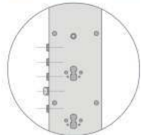
Vers. D : 4 Pistoni int. 28 + scrocco + blocca-aste Type D : 4 Bolts int. 28 + latch bolt + bar stopper
