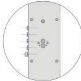
Vers. A : 4 Pistoni int. 28 + scrocco Type A : 4 Bolts int. 28 + latch bolt
