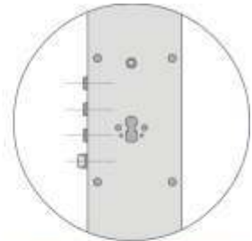
Vers. B : 3 Pistoni int. 37 + scrocco Type B : 3 Bolts int. 37 + latch bolt
