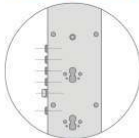
Vers. C : 4 Pistoni int. 28 + scrocco + blocca-aste Type C : 4 Bolts int. 28 + latch bolt + bar stopper
